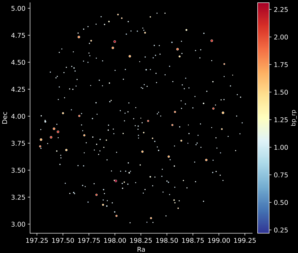
GALAH DR4 Field: [9336] Stars: 272
