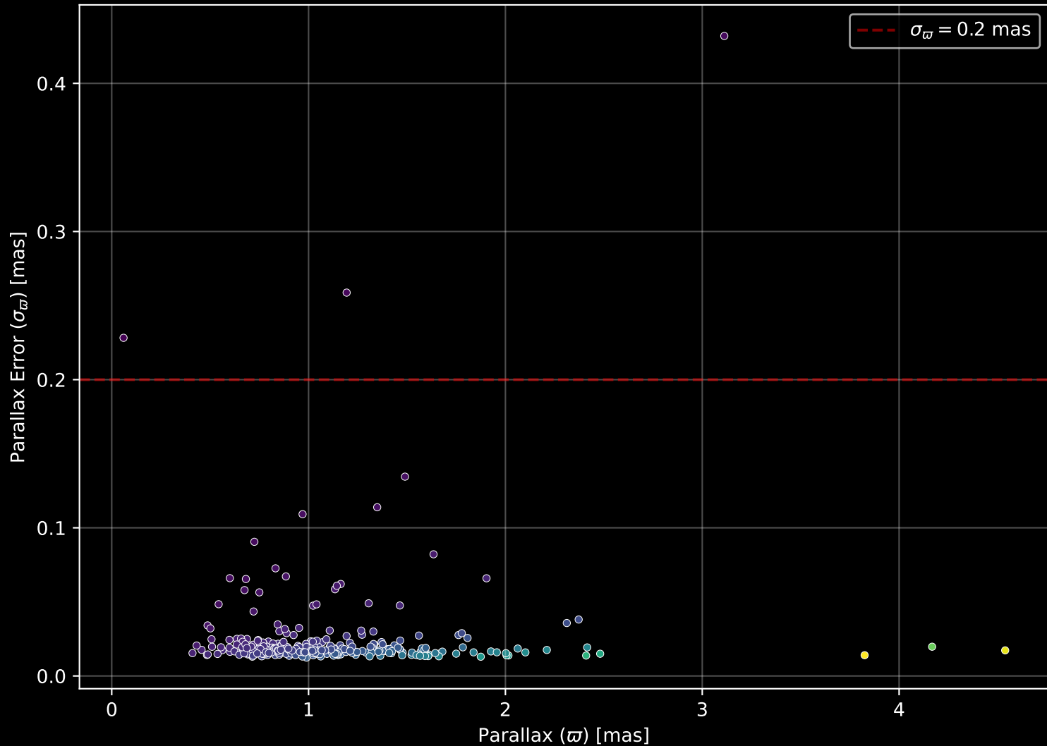
GALAH DR4 Field: [9336] Parallax Quality (n= 272)
