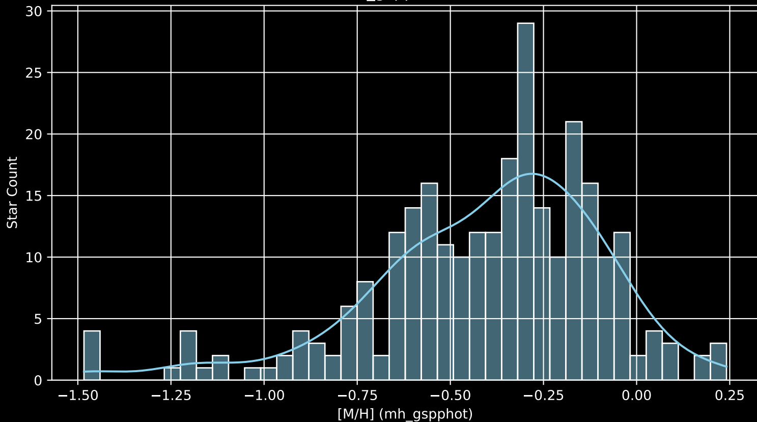
GALAH DR4 Field: [9336] [M/H] (mh_gspphot) (n= 272)
