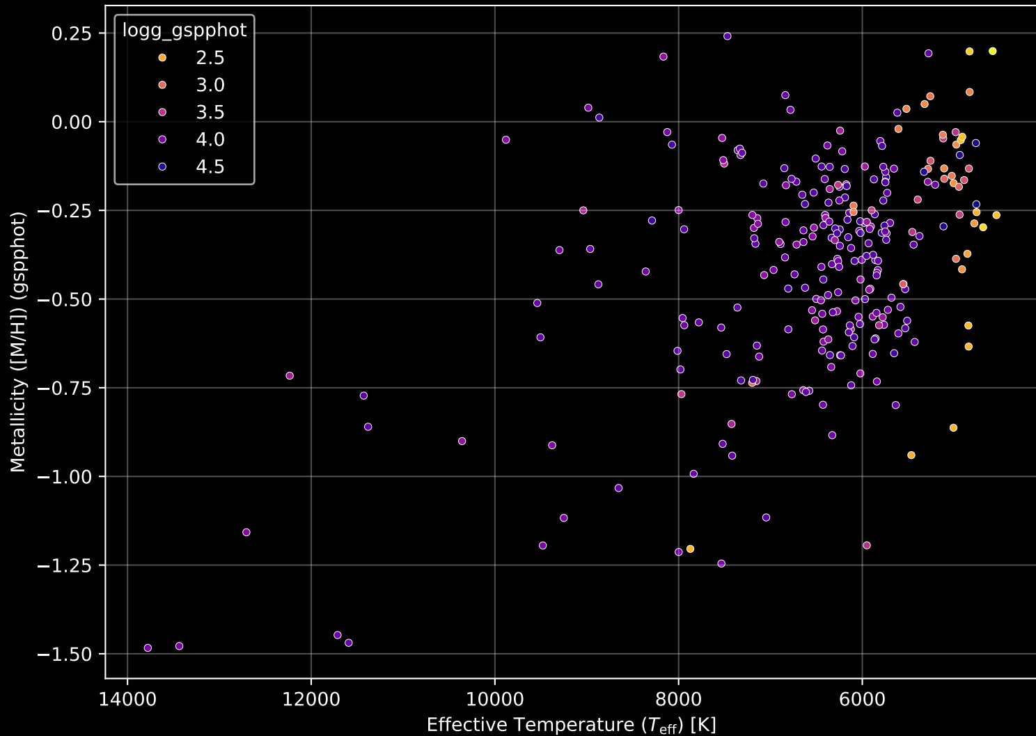
GALAH DR4 Field: [9336] Stellar Population Parameters (n= 272)
