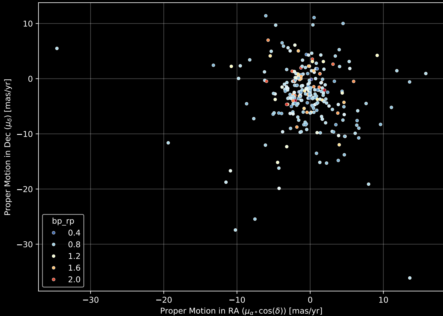
GALAH DR4 Field: [9336] Proper Motion Diagram (n= 272)
